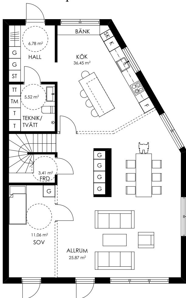
Entréplan
